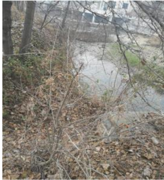
河道右岸、紧靠交通桥处挡墙坍塌
